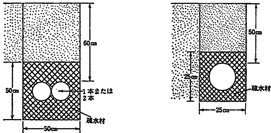
吸水管理埋設図
