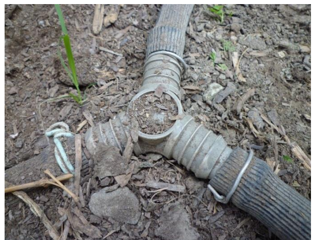
図3 図2の接続部を掘り起こした写真
