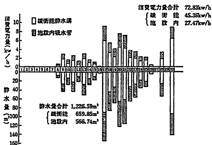
図 9 消費電力および地下排水（50 年 4 月）
