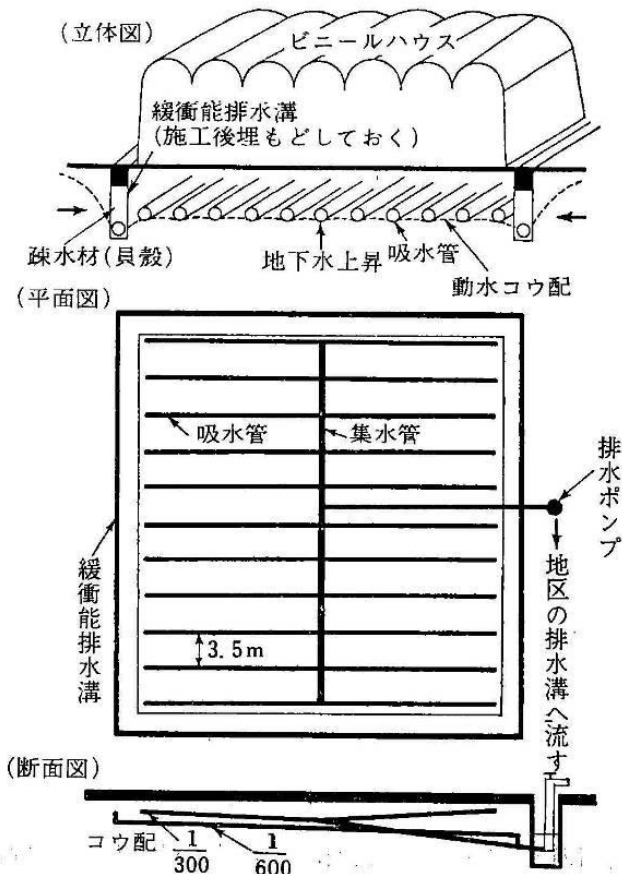
図2 地下水位制御装置
