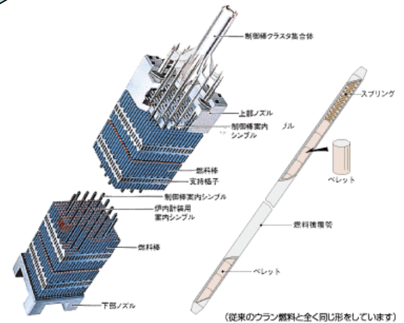
燃料集合体と制御棒クラスタ
