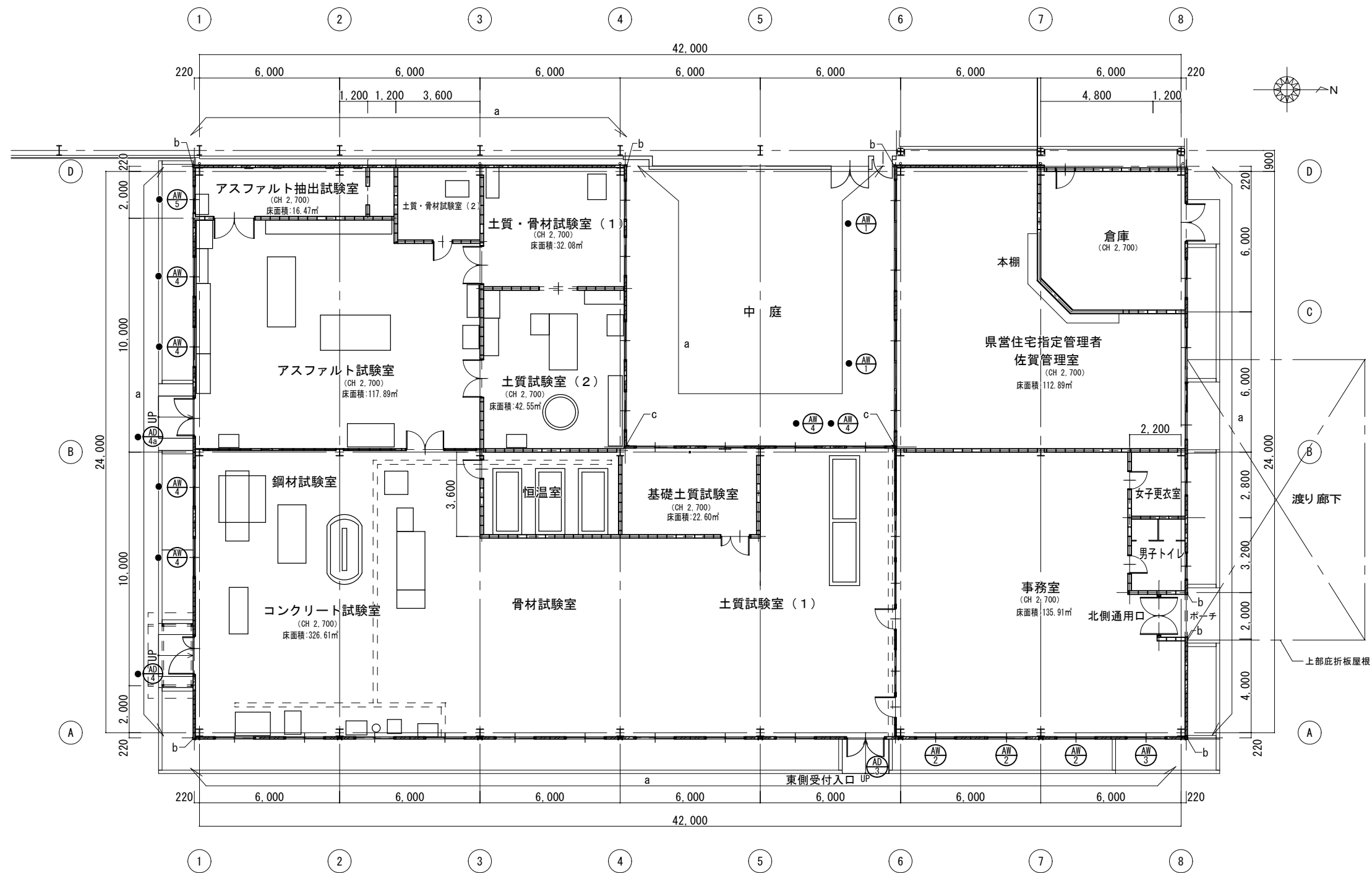
平面図 S:1/100
