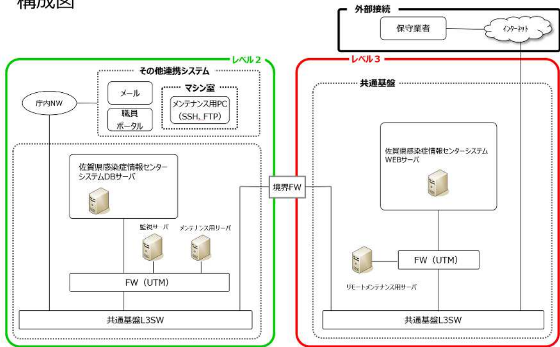
図 1 ハードウェア・ネットワーク構成図
