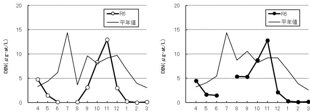
図 7 DINの推移 (10定点平均値, 左図: 表層, 右図: 底層)
