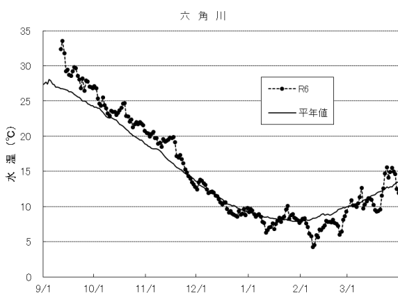
図17 水温の推移（六角川自動観測塔）
