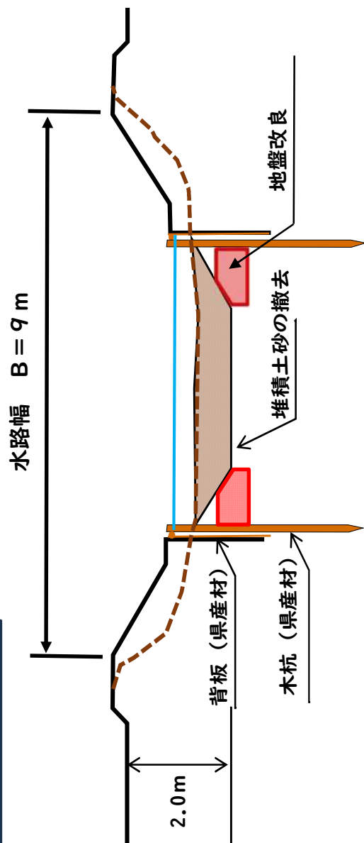
標準断面図
