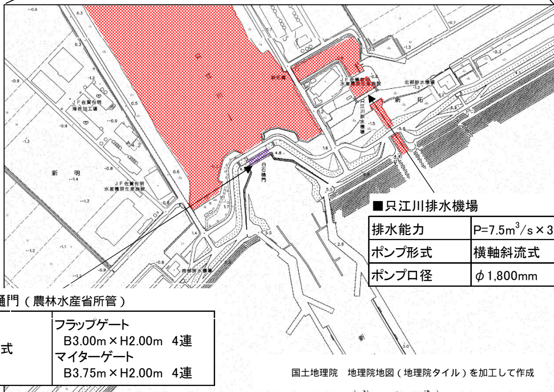
図6 平面図
