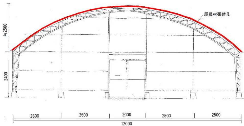
図4. 立面図
