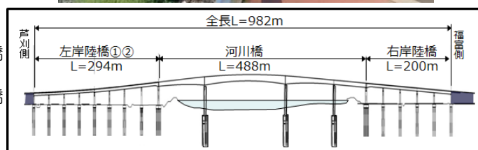
【河川橋】橋長488m 構造:4径間連続鋼床版箱桁橋
