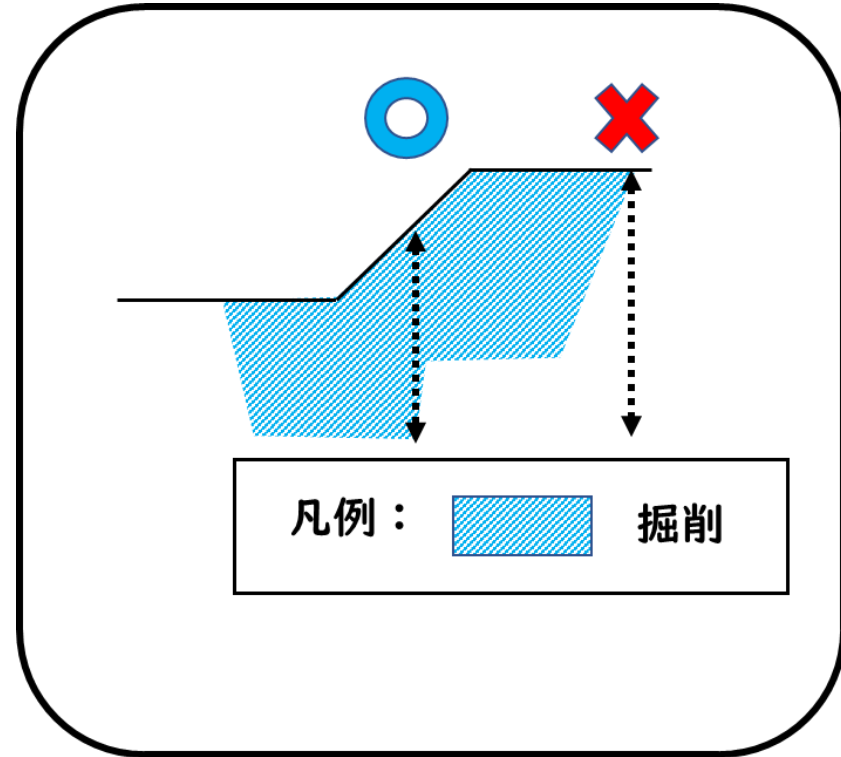
例2:斜面を掘削する場合の掘削深度
