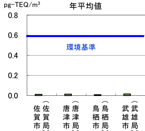
図 2-2-47 大気環境中のダイオキシン類濃度 資料：環境課
