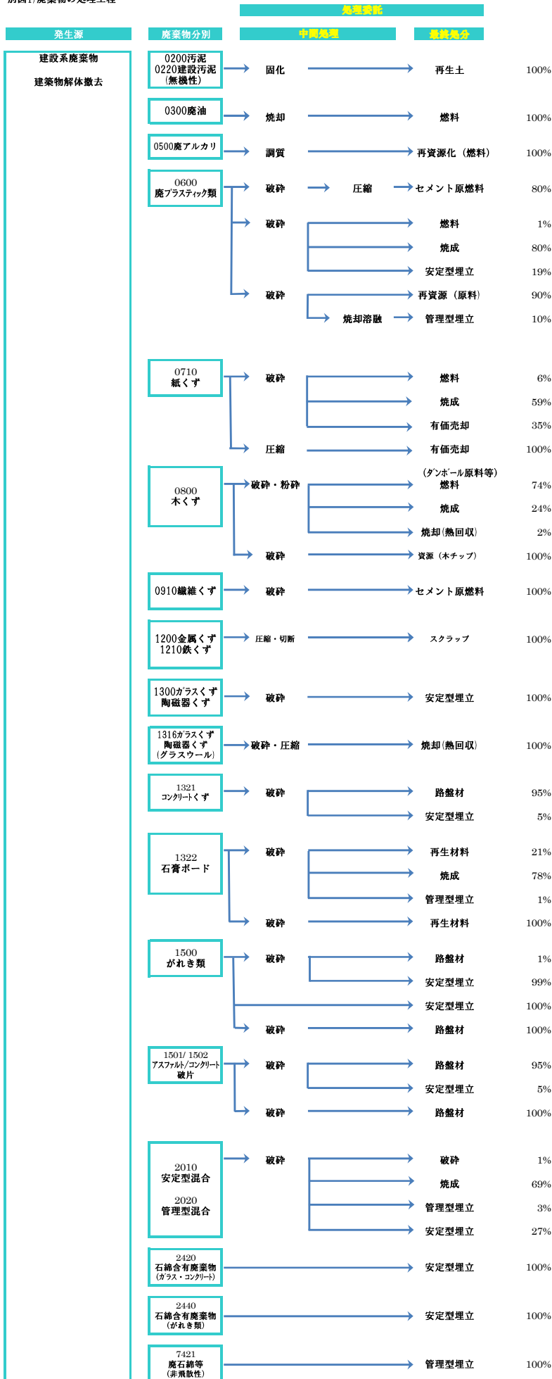
別図1) 廃棄物の処理工程
