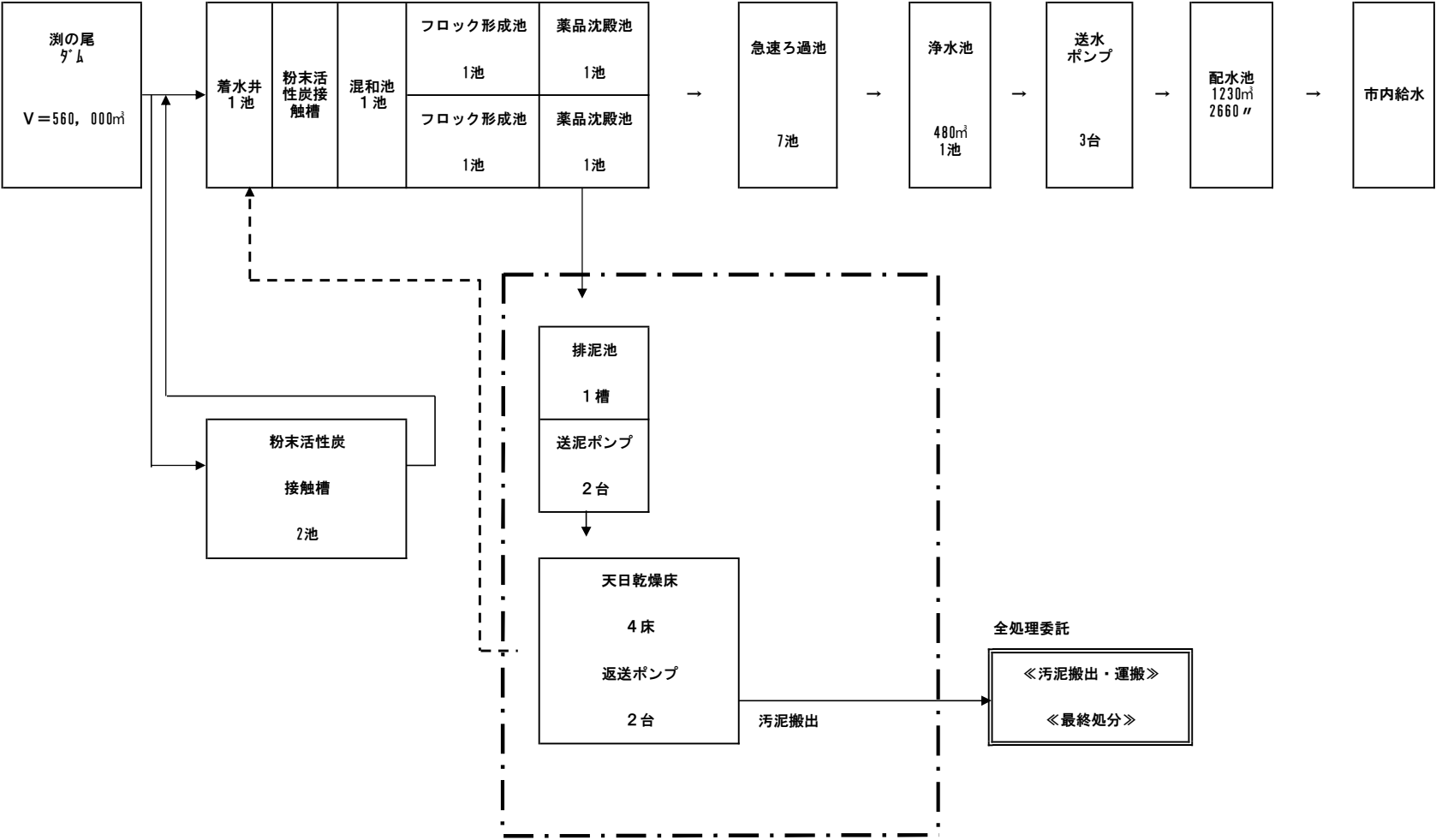
淵の尾浄水場フローシート<図-1>
