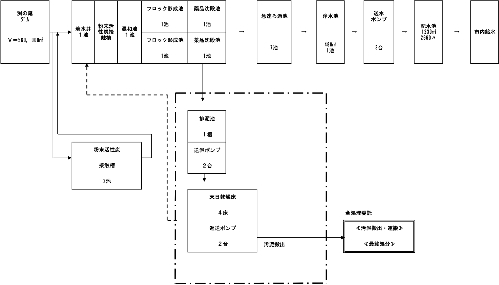
淵の尾浄水場フローシート<図-1>
