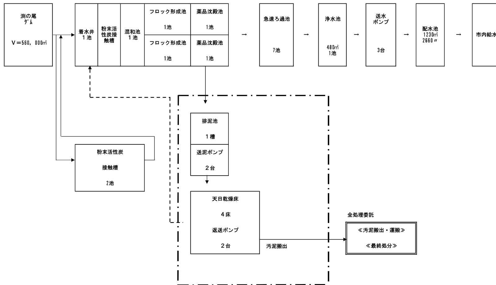
渚の尾浄水場フローシート<図-1>
