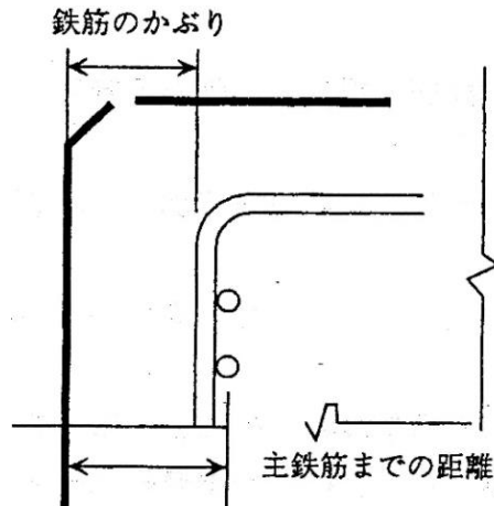
図 6-1 鉄筋のかぶり
