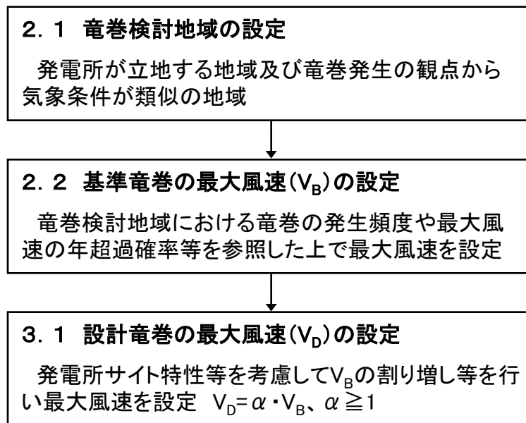
図2.1 設計竜巻の設定フロー
