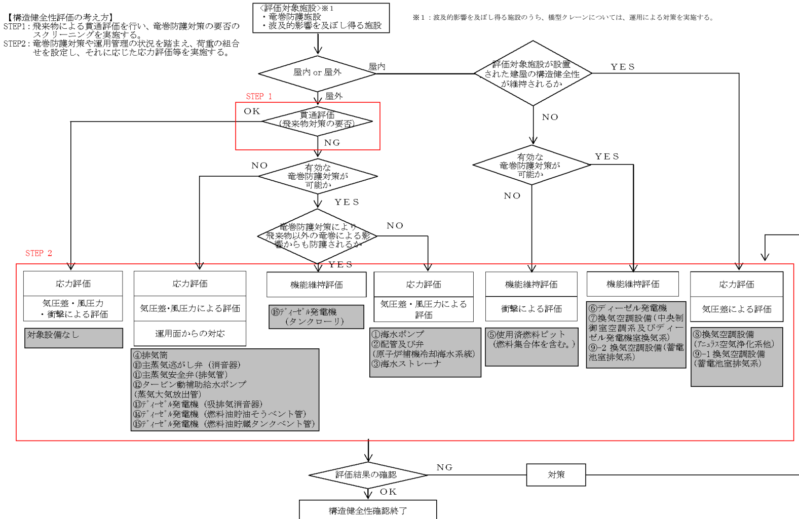
図6.4 竜巻防護施設及び竜巻防護施設に波及的影響を及ぼし得る施設(設備)の構造健全性評価フロー
