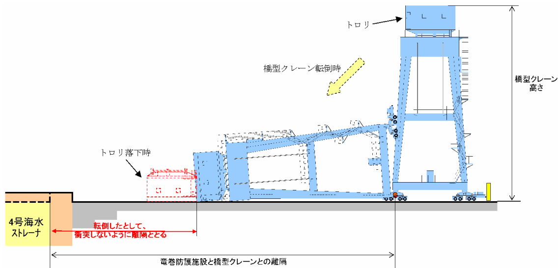
図7.11 橋型クレーン転倒時のイメージ図
