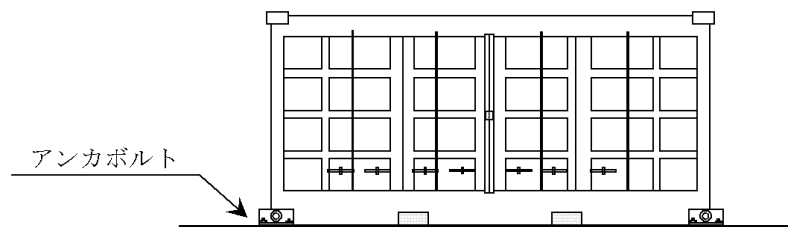
図7.2 コンテナの固定(例)
