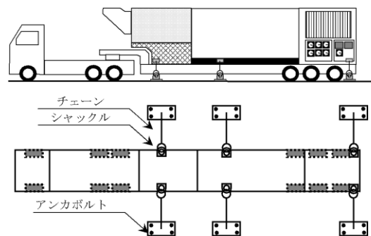
図7.1. 車両の固縛
