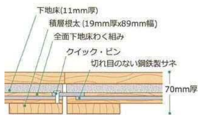
組み立てのための取り付け部品
