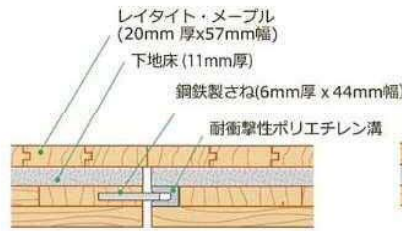
サネ継ぎ詳細図
