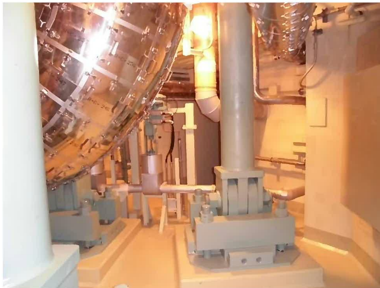
蒸気発生器支持構造物点検
