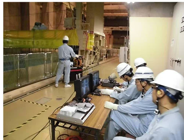
使用済燃料ピットラックセル点検(撮影映像確認)
