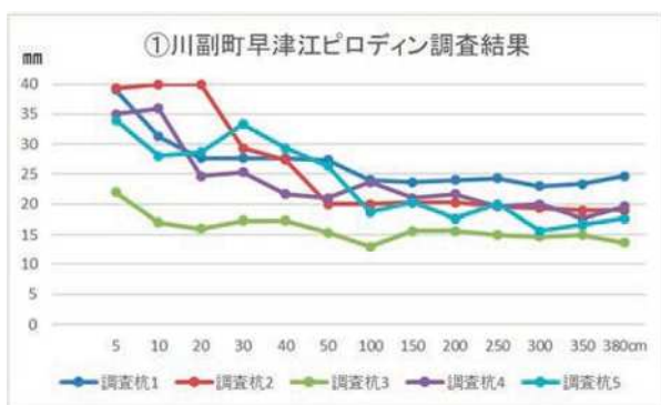
図-1-1 調査地①のピロディン貫入深度
