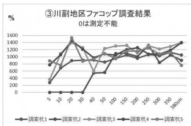
図一 2－3 調査地③の応力波伝播速度
