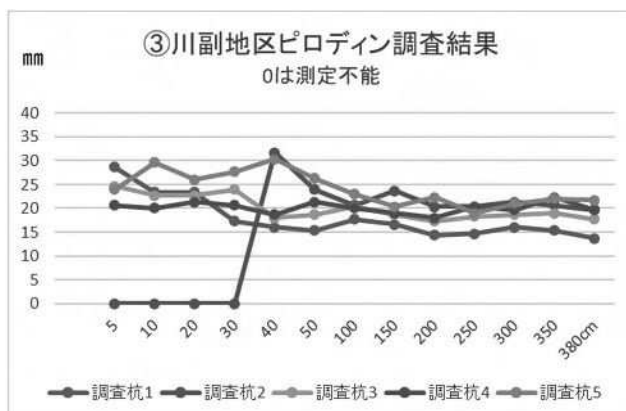
図－1－3 調査地③のピロディン貫入深度
