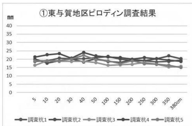
図－1－1 調査地①のピロディン貫入深度
