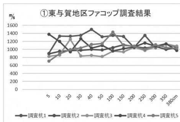
図－2－1 調査地①の応力波伝播速度
