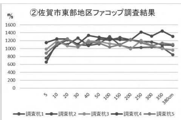
図－2－2 調査地②の応力波伝播速度
