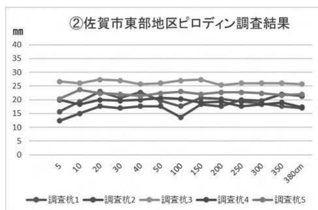
図－1－2 調査地②のピロディン貫入深度
