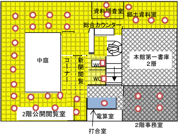
二階平面図
