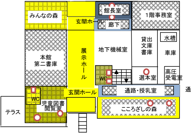
一階平面図
