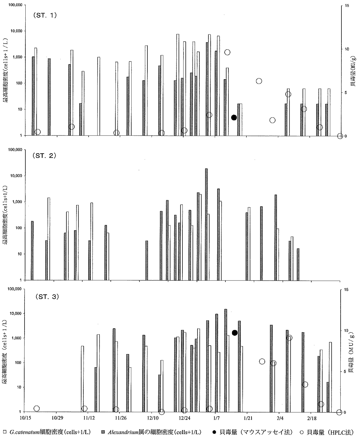
図5 Alexandrium 属と G. catenatum の最高細胞密度 (cells/L) と貝毒量 (MU/g) の推移
