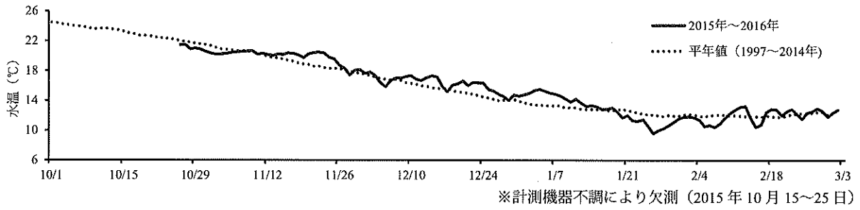
図3 2015年10月～2016年3月における記録式水温計による水温連続観測（水深2 m）
