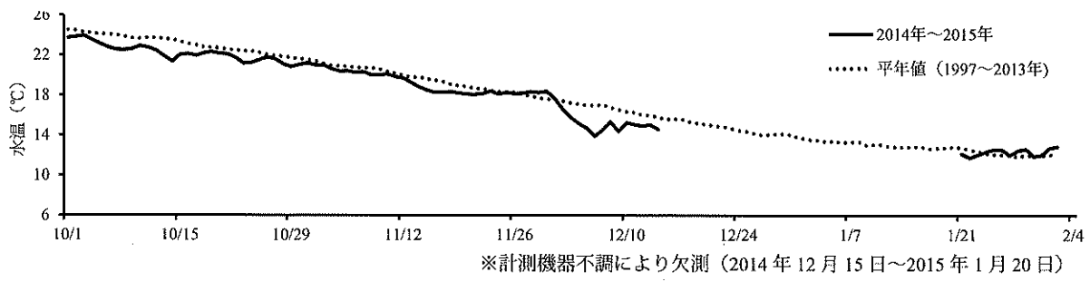
図3 2014年10月～2015年2月における記録式水温計による水温連続観測（水深2 m）
