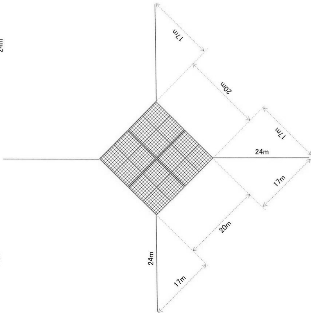
水平図
