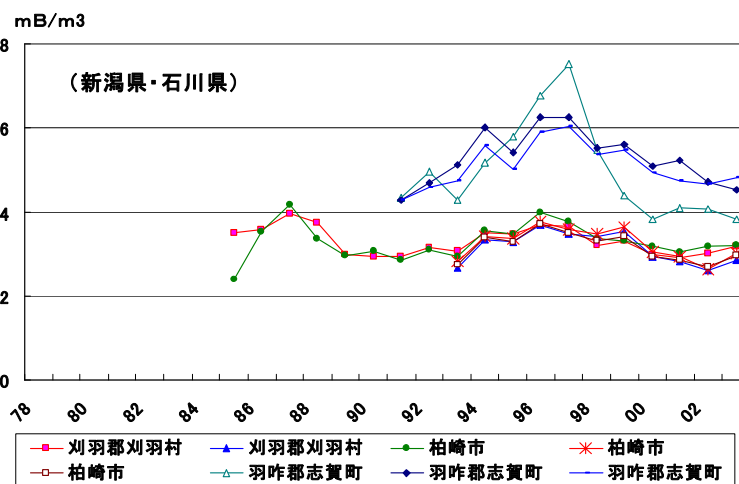
図4-1 浮遊粉じん中 7 Be 月間値の年平均値グラフ
