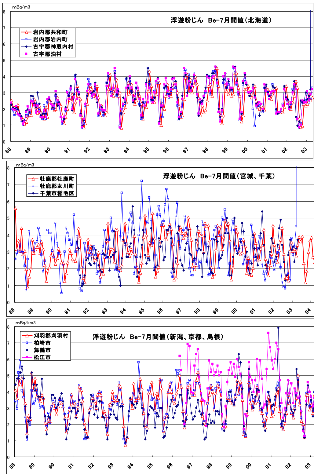
図3 浮遊粉じん中 ^7\text{Be} 月間値の挙動
