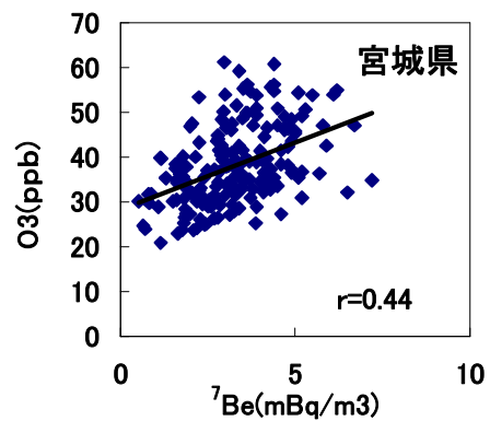
浮遊粉じん 7 Be 月間値とオゾン月平均値の相関
