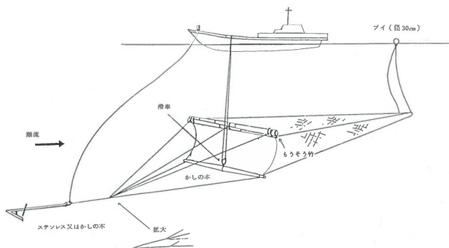
図1 あんこう網漁業の構造図
