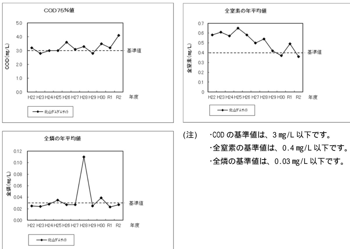
図 2-2-28 北山ダム COD75%値、全窒素年平均値、全燐年平均値の推移 資料：環境課
