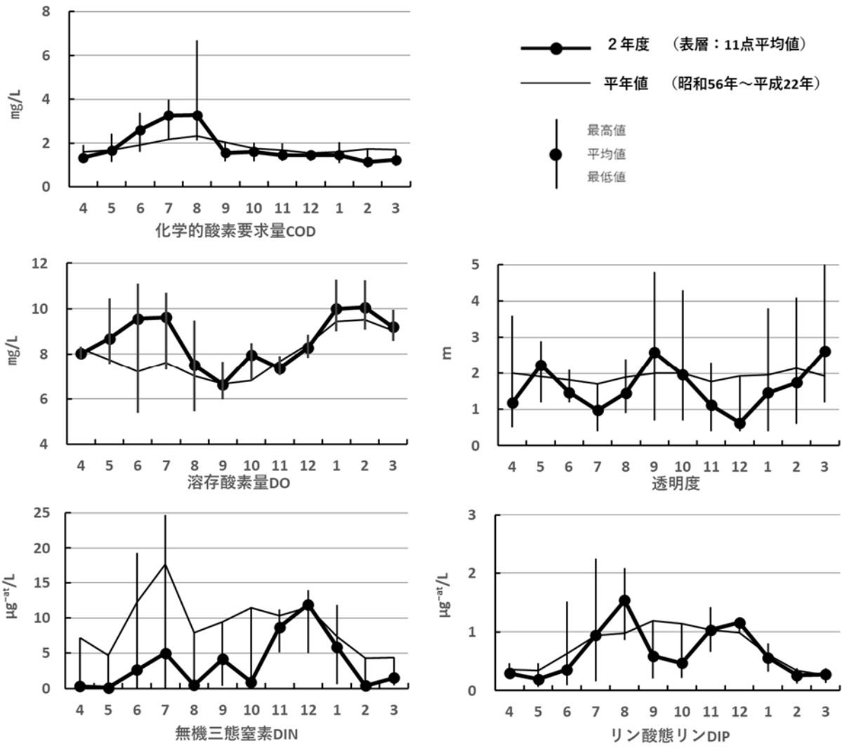
図 2-2-37 有明海の漁場の水質調査結果（令和 2 年度）
