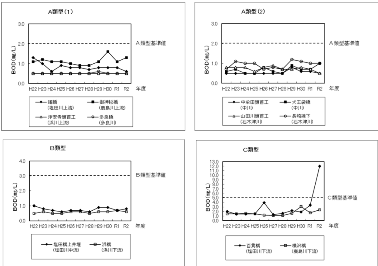
図 2-2-27 塩田川水系 BOD75%値の推移
