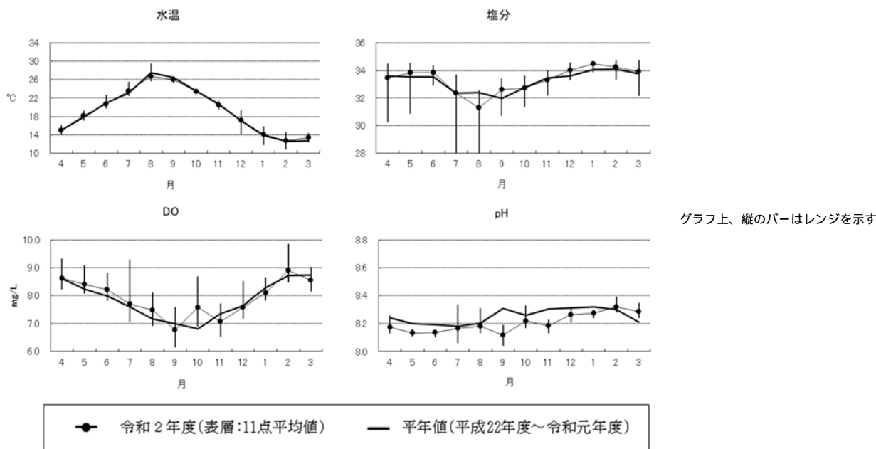
図2-2-39 玄海漁場環境保全調査結果(表層)(令和2年度)
