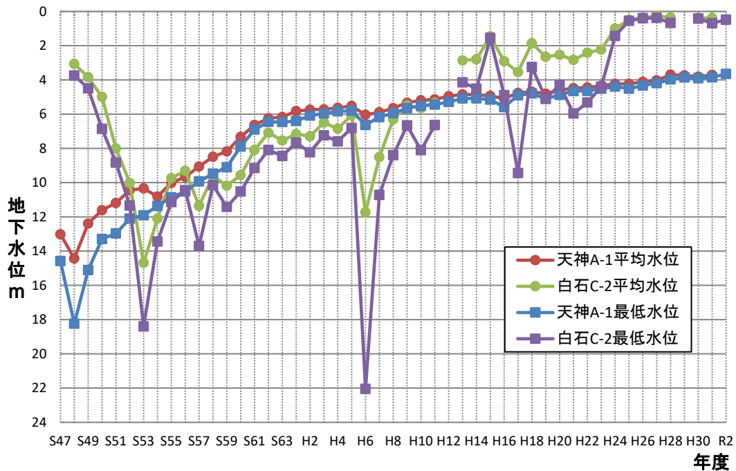
図2-2-43 代表的な観測井の地下水位の経年変化
