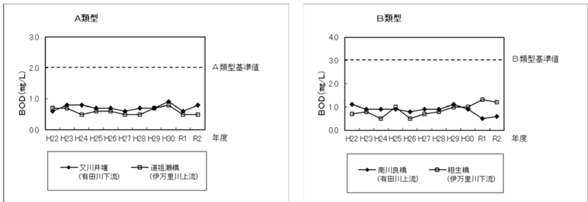
図 2-2-26 有田・伊万里川水系 BOD75%値の推移
