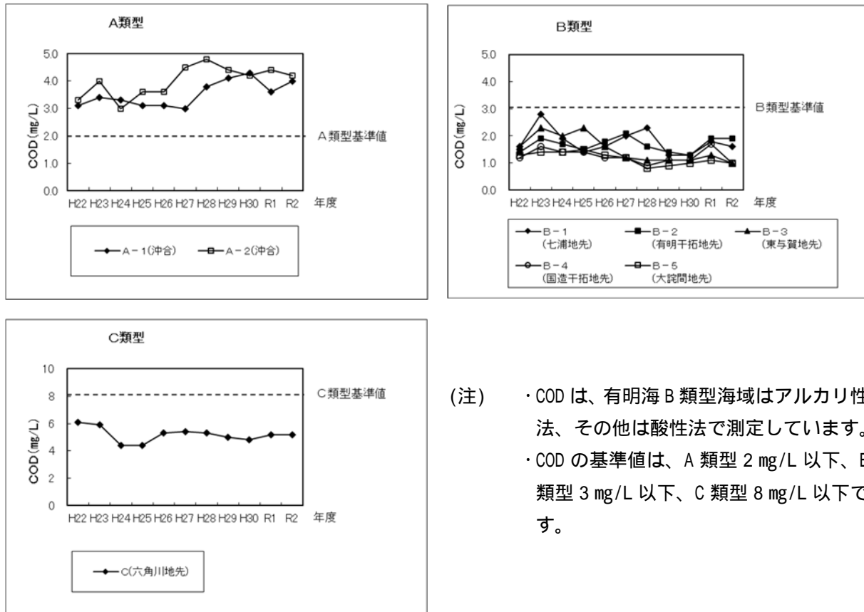
図 2-2-29 有明海海域 COD75%値の推移
