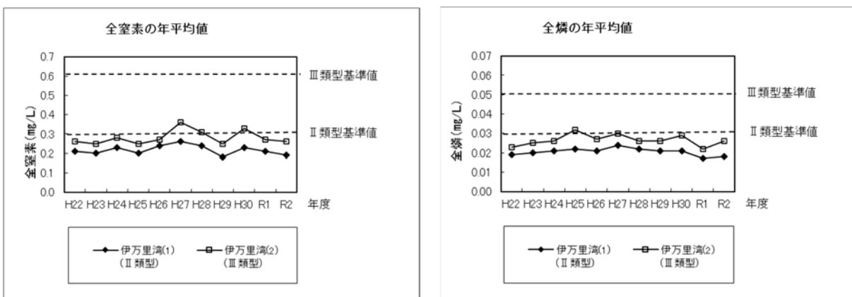
図 2-2-33 伊万里湾 全窒素・全磷の年平均値の推移
