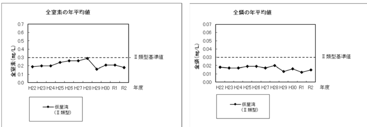
図 2-2-34 仮屋湾 全窒素・全磷の年平均値の推移
