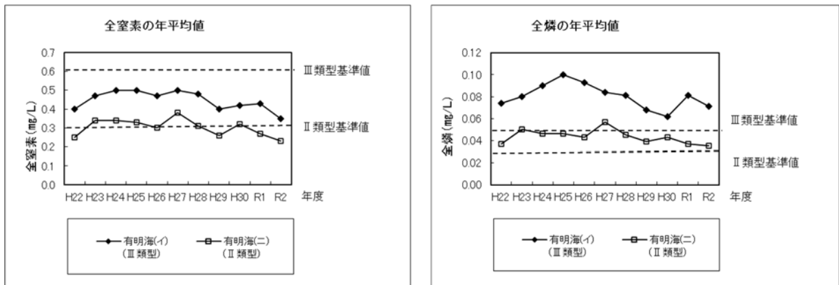
図 2-2-30 有明海海域 全窒素・全燐の年平均値の推移
