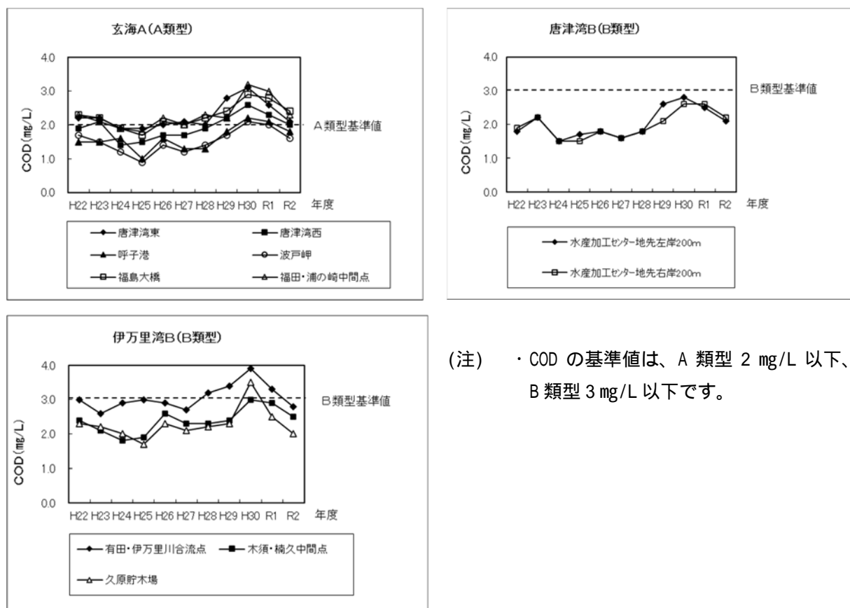
図 2-2-31 玄海海域 COD75%値の推移
