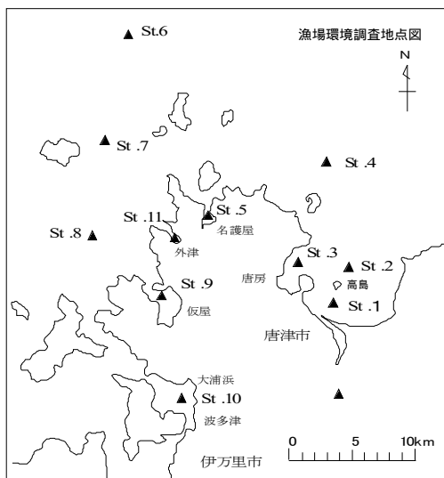
図2-2-38 玄海海域漁場環境調査定点(令和2年度)
