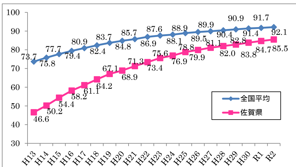
図 2-2-40 汚水処理人口普及率推移表 資料：下水道課
