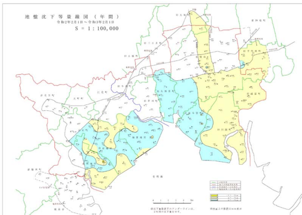
図2-2-41 地盤沈下等量線図（年間）
