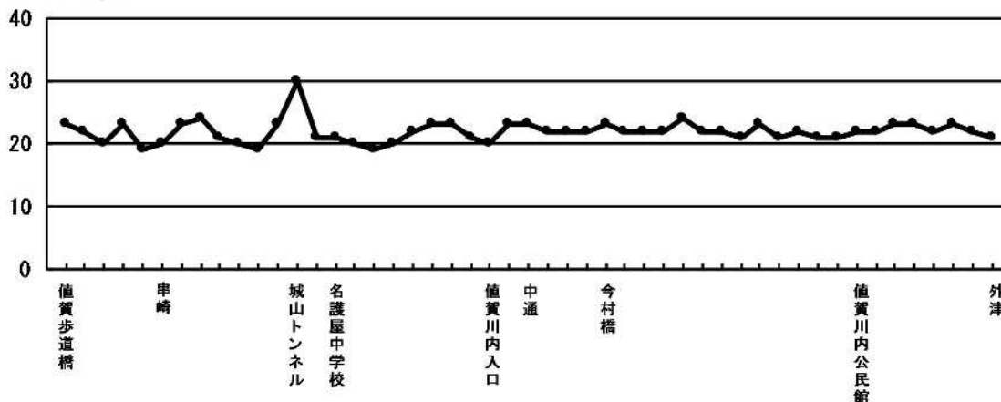
線量率 (nGy/h)
