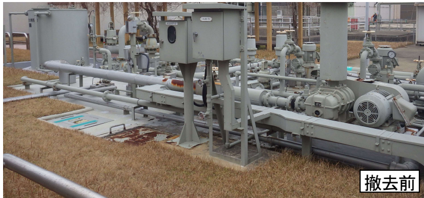
復水脱塩装置(中和槽・排水槽排水設備)
